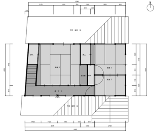
各務原市 那加大平町 2F 平面図
