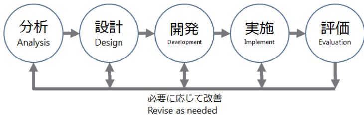
図 1 – 1 ADDIE モデル
