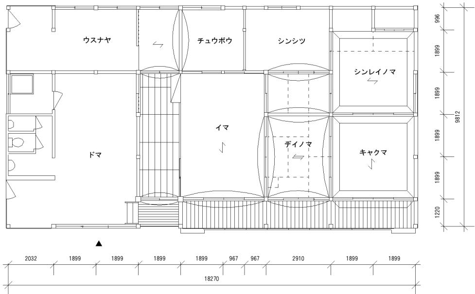
平面図 S=1:150
