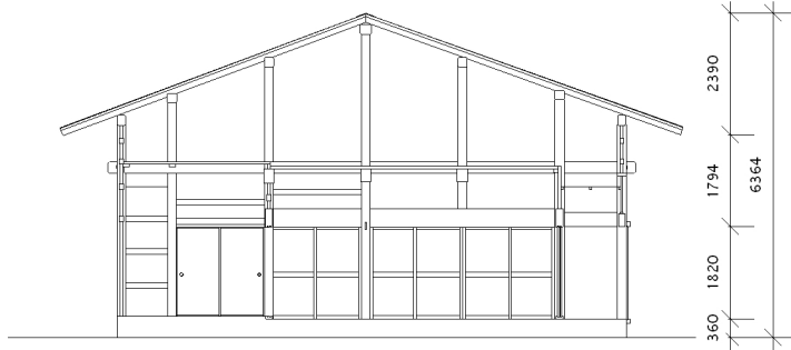
梁間断面図 S=1:150
