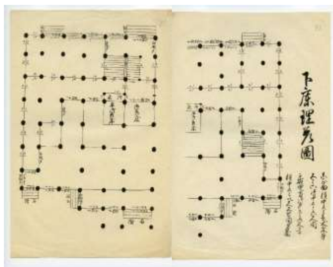
図2 百浦添御殿普請付御絵図并御材木寸法記(下庫理差図)
